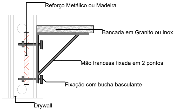
DETALHE 01: REFORÇO EM DRYWALL
